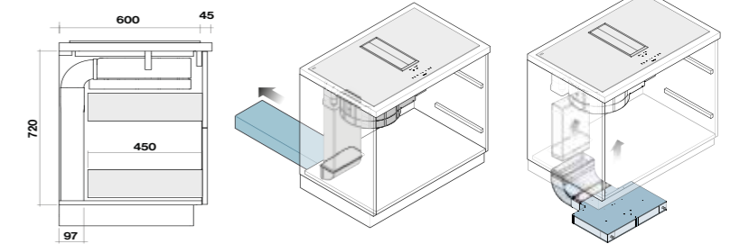
Installation i 60cm bordplade og større end.
