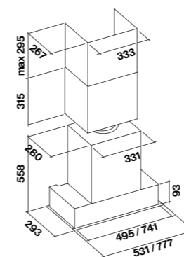
Udskæringsmål 60 cm: 506 mm x 262 mm 80 cm: 751 mm x 262 mm
