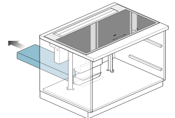
Løsning med aftræk Sokkelhøjde minimum 100 mm
