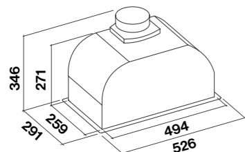
Udskæringsmål 50 cm: 506 mm x 262 mm 70 cm: 751 mm x 262 mm
