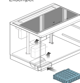
Recirkulations-løsning Kulfilter type 930 Sokkelhøjde minimum 100 mm
