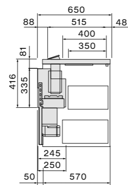
Fra siden Installation i min. 65cm bordplade
