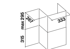
Optional chimney
