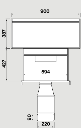
Brooklyn Μπροστινή όψη
