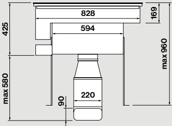
Πλάγια όψη με το μοτέρ τοποθετημένο μπροστά
