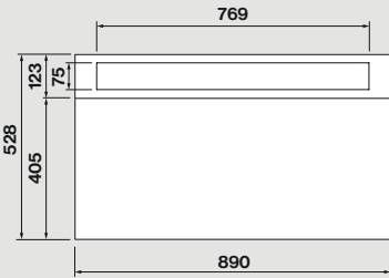
Άνω όψη
