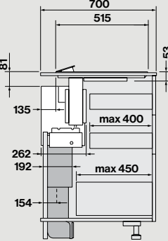
Πλάγια όψη με το μοτέρ τοποθετημένο πίσω με το Kit Silence KACL.1026
