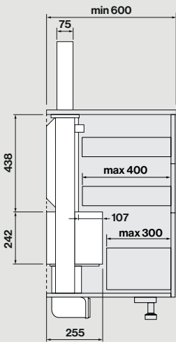
Πλάγια όψη με το μοτέρ τοποθετημένο μπροστά
