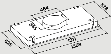
Μοτέρ Slim (μόνο πάνω στον απορ/ρα)
