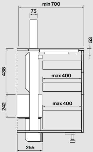
Πλάγια όψη με το μοτέρ τοποθετημένο πίσω
