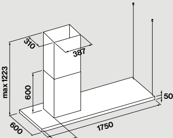
Versione sinistra
