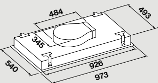
Μοτέρ Slim (μόνο πάνω στον απορ/ρα)
