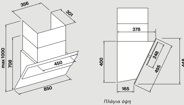
Πλάγια όψη
