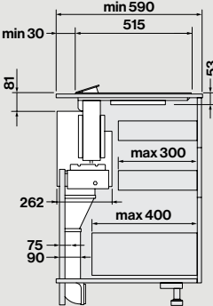
Πλάγια όψη με το μοτέρ τοποθετημένο μπροστά
