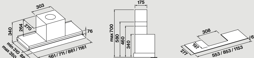
Πλάγια όψη con Προαιρετική καμινάδα
