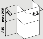
Προαιρετική καμινάδα
