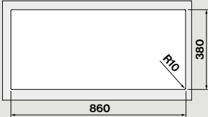
Διαστάσεις τρύπας
