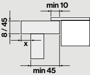
Διαστάσεις τρύπας
