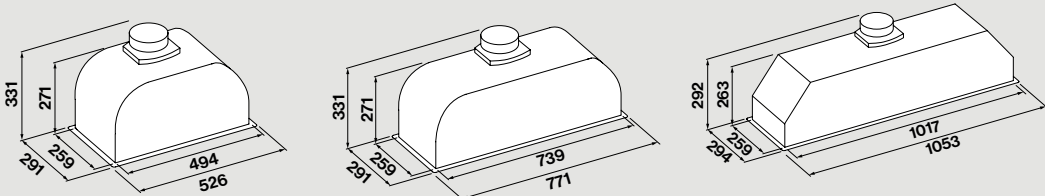
Τρύπα εντοιχισμού 50 cm: 262 x 506 mm 70 cm: 262 x 751 mm
