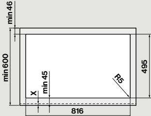
Διαστάσεις τρύπας
