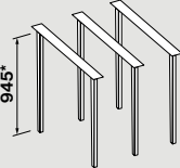
KACL.748#IF KACL.748#HF *Μέγιστο ύψος με κιτ επέκτασης δοκών: 1550 mm.
