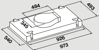
Μοτέρ Slim (μόνο πάνω στον απορ/ρα)
