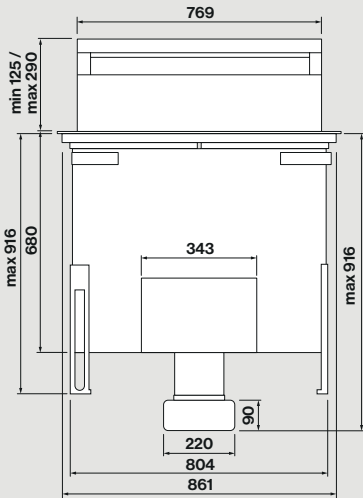
Μπροστινή όψη
