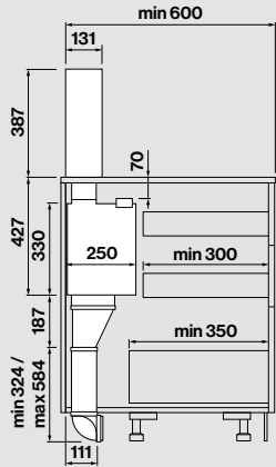
Παράδειγμα διαμόρφωσης Πλάγια όψη με το μοτέρ τοποθετημένο μπροστά
