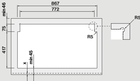
Διαστάσεις τρύπας
