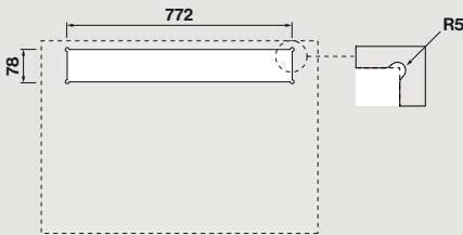
Διαστάσεις τρύπας
