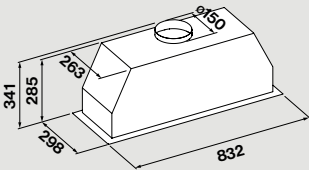
Τρύπα εντοιχισμού 267 x 807 mm
