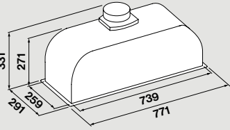
Τρύπα εντοιχισμού 50 cm: 262 x 506 mm 70 cm: 262 x 751 mm
