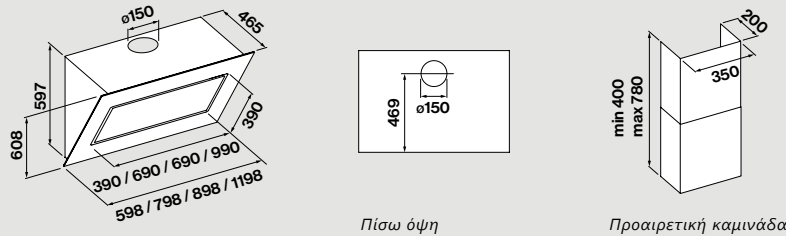
Πίσω όψη Προαιρετική καμινάδα
