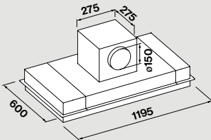
Μοτέρ τετράγωνο τοποθετημένο πάνω στον απορ/ρα
