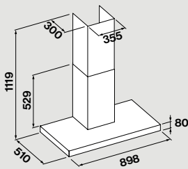
Τοίχου
