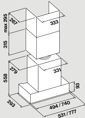
Τρύπα εντοιχισμού 50 cm: 262 x 506 mm 70 cm: 262 x 751 mm
