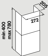
Προαιρετική καμινάδα
