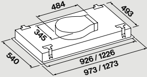
Απομακρυσμένα μοτέρ
