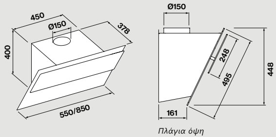
Πλάγια όψη
