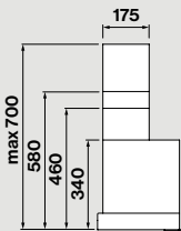
Πλάγια όψη con Προαιρετική καμινάδα
