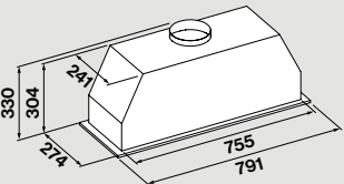
Τρύπα εντοιχισμού 245 x 762 mm
