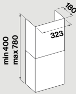
Προαιρετική καμινάδα
