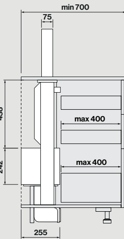
Πλάγια όψη με το μοτέρ τοποθετημένο πίσω
