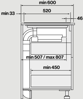
Πλάγια όψη
