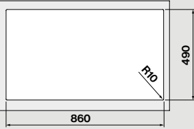
Διαστάσεις τρύπας
