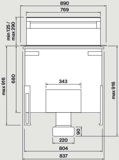
Πλάγια όψη με το μοτέρ τοποθετημένο μπροστά
