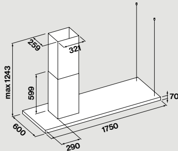
Περιοχή απορρόφησης 90 cm στην πλευρά της καμινάδας
