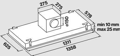
Μοτέρ τετράγωνο τοποθετημένο πάνω στον απορ/ρα
