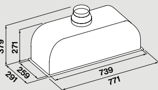
Τρύπα εντοιχισμού 50 cm: 506 mm x 262 mm 70 cm: 751 mm x 262 mm
