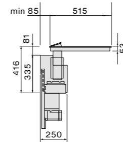
Vista laterale
