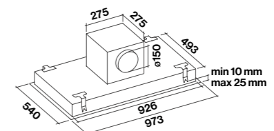
Raccordo (KACL.789)
