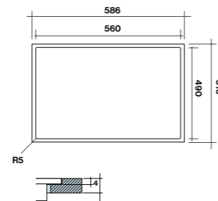
Dimensioni foro per installazione a filo
