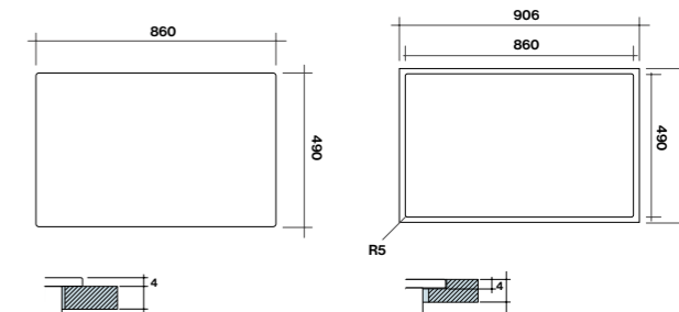
Dimensioni foro per installazione in appoggio
