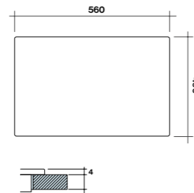
Dimensioni foro per installazione in appoggio
