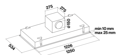
Raccordo (KACL.789)
