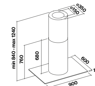
Versione Isola con vetro (opzionale)
