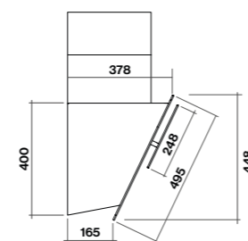
Vista laterale
