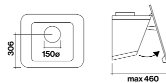
Vista posteriore
