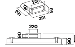
Raccordo (KACL.789)
