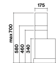
Vista laterale con camini opzionali
