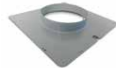
Flangia per motori e aspiratori ad alta potenza (1500 - 1300 m 3 /h) KACL.396 ø200 KACL.398 ø150
