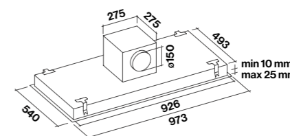
Raccordo (KACL.789)
