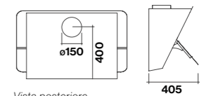
Vista posteriore
