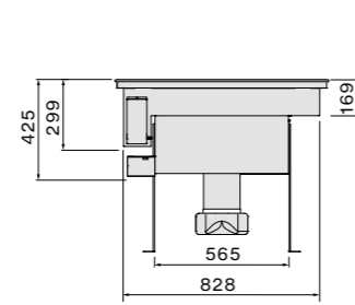
Vista frontale
