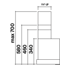
Vista laterale con camini opzionali
