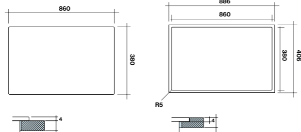
Dimensioni foro per installazione in appoggio
