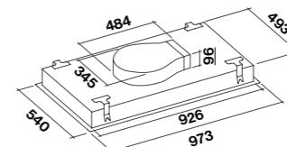
Motore sottotetto installato sulla cappa
