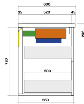
Vista laterale
