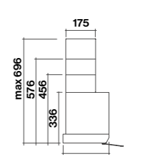
Vista laterale con camini opzionali
