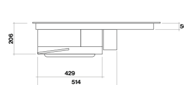
Vista frontale
