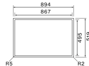
Foro di incasso Installazione a filo
