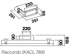
Raccordo (KACL.789)
