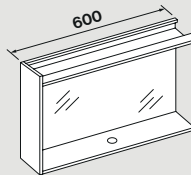
Rechtes/linkes Modul* mit Hahnloch (Ausschnitt Ø 35mm)
