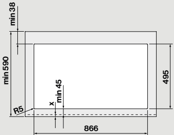
Ausschnittmaß
