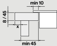
Ausschnittmaß
