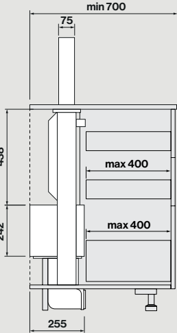
Seitenansicht mit Motor in Heckstellung
