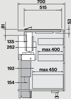
Seitenansicht mit Motor in Heckstellung mit Silence Kit 103076
