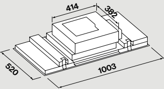
Ausschnitt 502 x 985 mm
