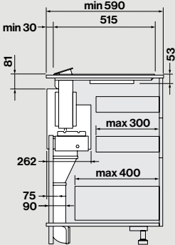
Seitenansicht mit Motor in Frontstellung
