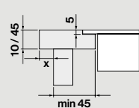
Flächenbündig
