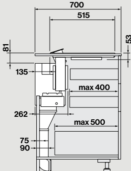
Seitenansicht mit Motor in Heckstellung
