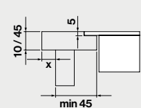
A filo
