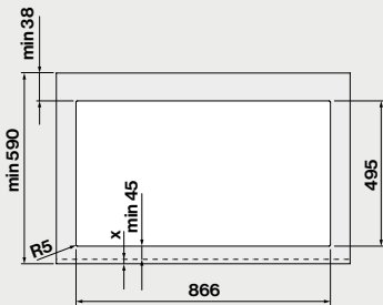
Dimensioni foro
