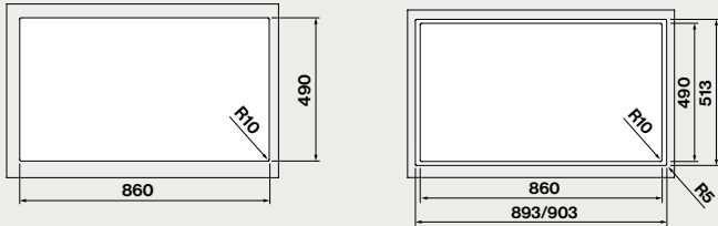
Dimensioni foro
