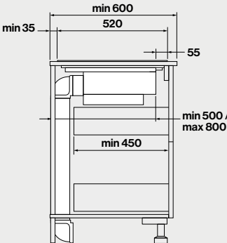
Vista laterale
