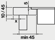
A filo
