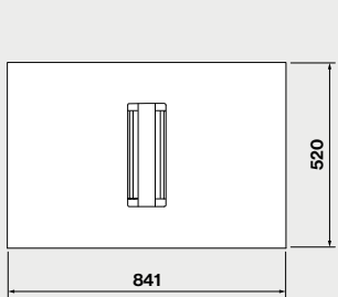
Vista superiore
