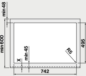
Dimensioni foro
