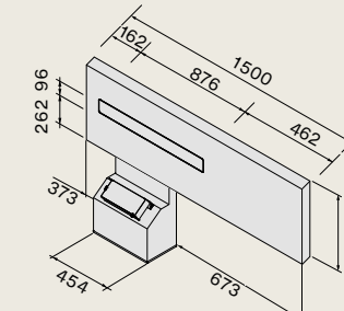
Air Wall 150 Ausführung 150 cm Absaugung links
