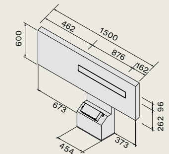
Air Wall 150 Ausführung 150 cm Absaugung rechts
