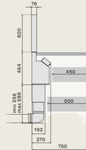
Air Wall versión con extracción Instalación en encimera profunda 75 cm Vista lateral
