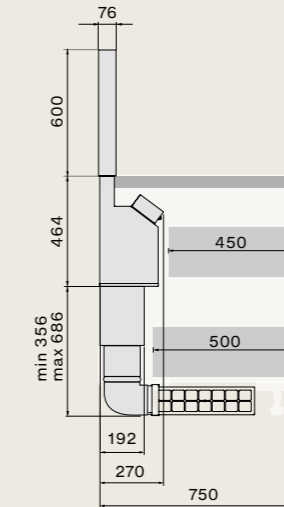
Air Wall versión con recirculación Instalación en encimera profunda 75 cm Vista lateral
