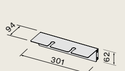
Accessoire met glazenhouder KACL.1025#HF
