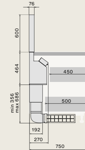
Air Wall recirculatie versie Aan de bovenzijde diepte 75 cm zijaanzicht
