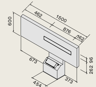
Air Wall 150 Module paneel 150 cm rechts afzuiging
