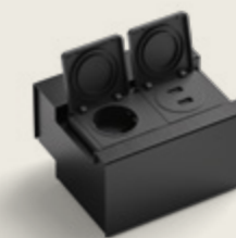
Prises électriques / usb L 147 x P 128 x H 86 mm
