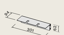
Accessoire met glazenhouder KACL.1025#HF
