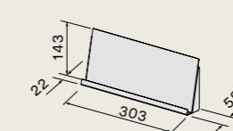
Accessoire rek voor boeken/tablets KACL.1024#HF
