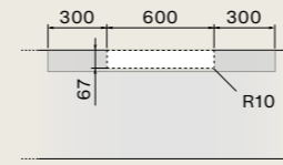
Air Wall afvoer versie aan de bovenzijde diepte 75 cm zijaanzicht
