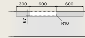
Air Wall recirculatie versie aan de bovenzijde diepte 75 cm zijaanzicht
