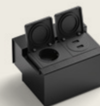
Розетки / Порты USB 147 × 128 × 86 мм (Д × Г × В)
