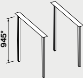
102536 *Maximale Höhe mit optionalen Verlängerungsstangen: 1550 mm.
