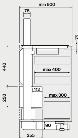
Seitenansicht mit Kanal Set 104187
