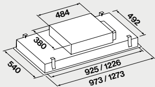
Ausschnitt 90 cm: 505 x 940 mm 120 cm: 505 x 1240 mm
