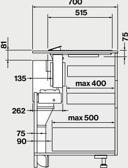
Seitenansicht mit Motor in Heckstellung (Inseleinbau)
