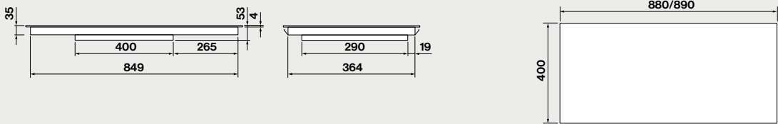
Frontansicht
