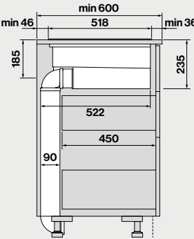
Seitenansicht mit Kanal Set 104172
