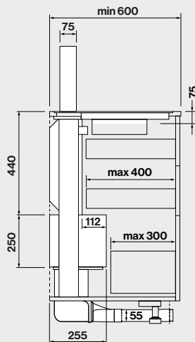
Seitenansicht mit Kanal Set 104188
