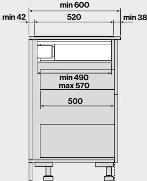
Seitenansicht mit mitgeliefertem Teleskoprohr
