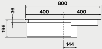
Frontansicht
