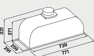
70 cm: 262 x 751 mm
