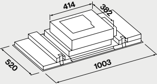
Ausschnitt 502 x 985 mm
