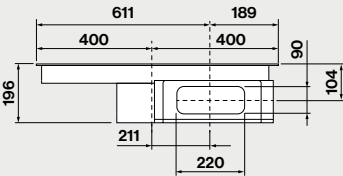
Rückansicht
