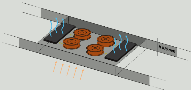
Multi-Air Filtration. 4 ultrakompakte Motoren und 2 Carbon.Zeo Filter
