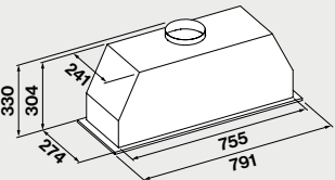
Ausschnitt 245 x 762 mm
