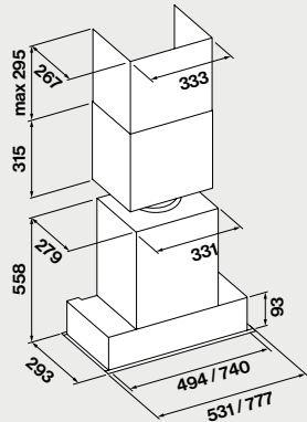
Ausschnitt 50 cm: 262 x 506 mm 70 cm: 262 x 751 mm
