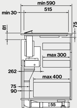
Seitenansicht mit Kanal Set 104188
