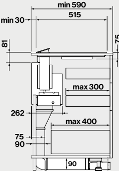
Seitenansicht mit Kanal Set 104187
