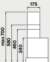
Seitenansicht mit optionalem Schacht
