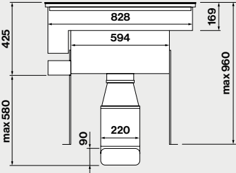
Seitenansicht mit Motor in Frontstellung (Wandmontage)
