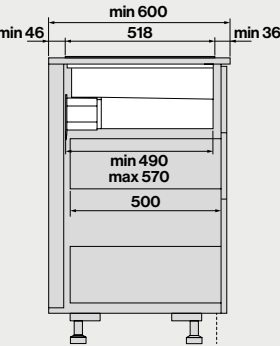
Seitenansicht mit mitgeliefertem Teleskoprohr
