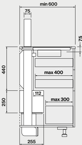
Seitenansicht mit Motor in Frontposition
