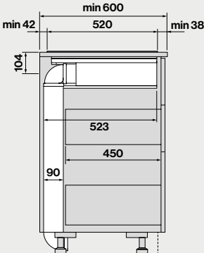
Seitenansicht mit Kanal Set 104172
