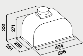
Ausschnitt 50 cm: 262 x 506 mm
