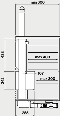
Seitenansicht mit Kanal Set 104188
