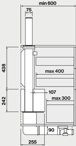
Seitenansicht mit Kanal Set 104187
