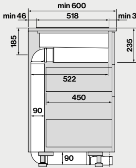
Seitenansicht mit Kanal Set 104174
