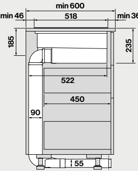
Seitenansicht mit Kanal Set 104173
