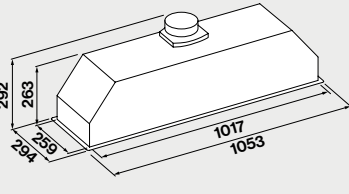
105 cm: 262 x 1029 mm
