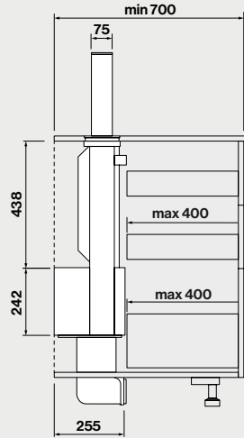
Seitenansicht mit Motor in Heckstellung
