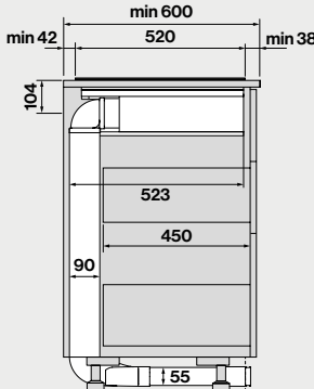
Seitenansicht mit Kanal Set 104173
