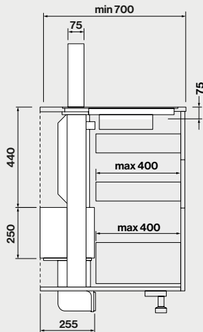
Seitenansicht mit Motor in hinterer Position
