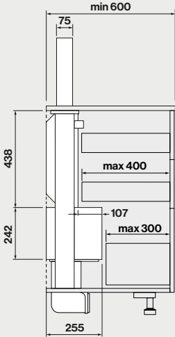
Seitenansicht mit Motor in Frontstellung
