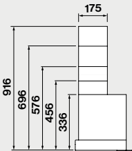
Seitenansicht mit optionalem Schacht
