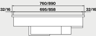
Frontansicht
