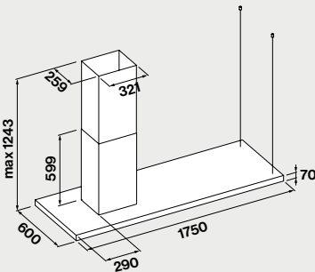
Absaugbereich 90 cm unter dem Schacht
