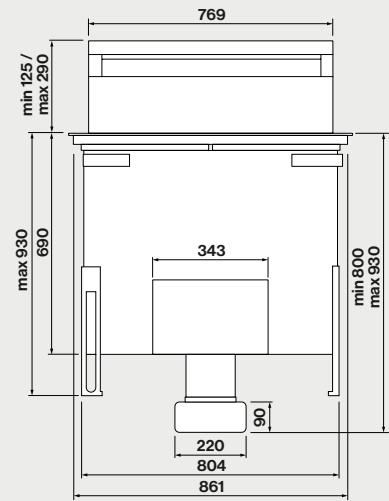
Seitenansicht mit Motor in Frontposition
