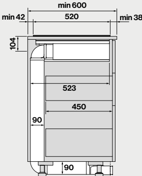
Seitenansicht mit Kanal Set 104174
